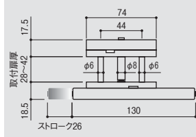
●外側引手部を外せば、内開き扉にも使用できます。
