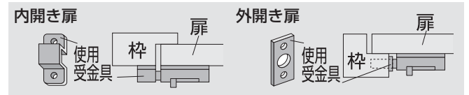
●外側引手部を外せば、内開き扉にも使用できます。
