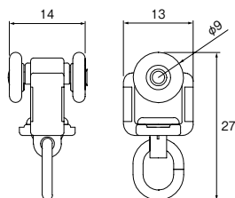
ランナー寸法図(単位: mm)
