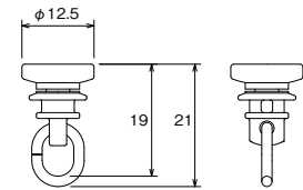
ランナー寸法図 (単位: mm)
