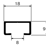
レール断面図 (単位: mm)
