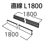
直線 L1800 本体 22 × 4.5 × 1800 ベース 23.3 × 4 × 1800
