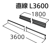
直線 L3600 本体 22 × 4.5 × 3600 ベース 23.3 × 4 × 1800
