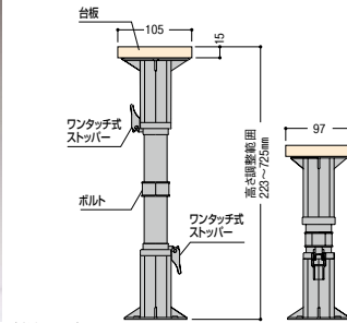
(単位:mm) 〈木造軸組工法の場合〉プラ束間隔・大引き間隔1000mm以内
