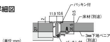
断面図
