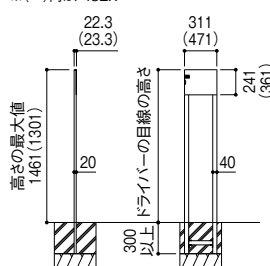
F33EX寸法図 (単位:mm) ※( )内はF48EX
