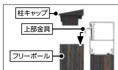
フリーポールに上部金具をかけます
