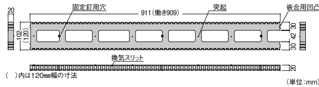
寸法図
