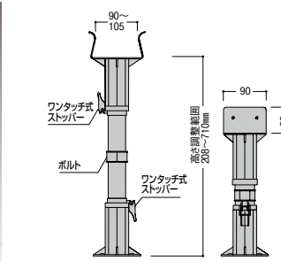
(単位:mm) 〈木造軸組工法の場合〉プラ束間隔・大引き間隔1000mm以内
