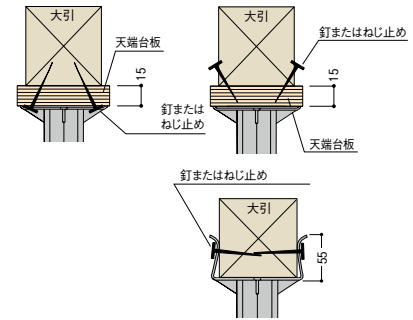
(単位:mm) 〈木造軸組工法の場合〉プラ束間隔・大引き間隔1000mm以内
