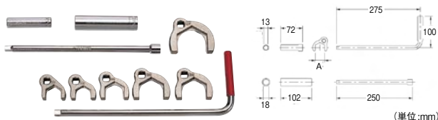
カクダイ 立形金具締めつけ工具セット
