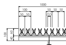
AGx詳細図
