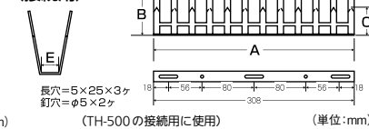
TH-308 (接続用)
