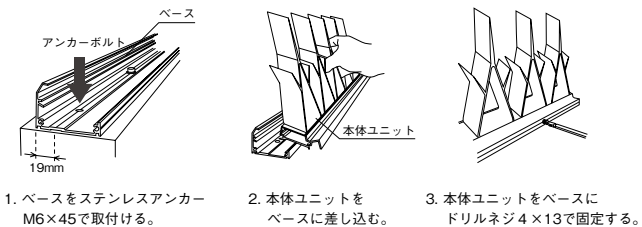
AGx詳細図
