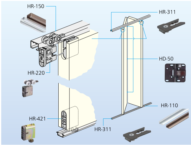
■金具の納まり参考図
