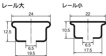
レール断面図
