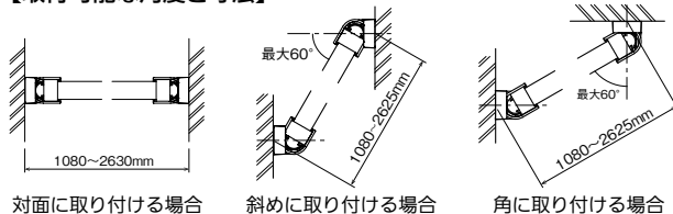
左右60°ずつ 首振り可能
