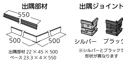
出隅部材 出隅部材 22 × 45 × 500 ベース 23.3 × 4 × 550
