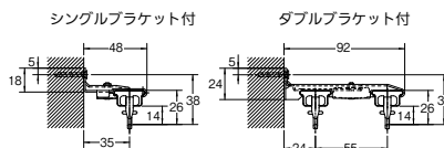
レール断面図
