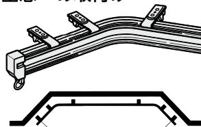
天井付シングルブラケット
