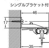
取付寸法図
