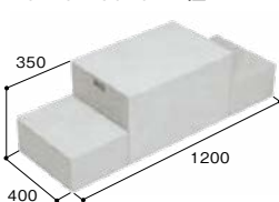
CUB-6040 1セット+ BU-CUB-6040D 1個
