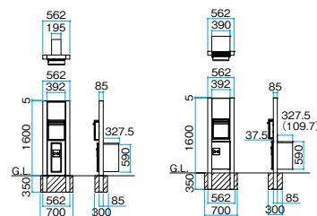
宅配ボックス：スリム
