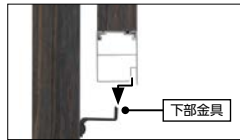
下部金具にフェンス本体をかけます
