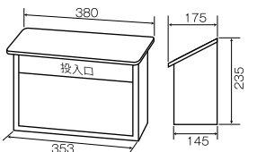
投入口サイズ: 318×38
