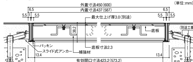
断面図 ( )内は600タイプを示します。
