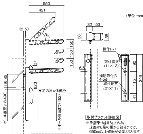
アーム角度 3段階
