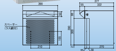
前入れ・後出し
