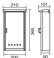
投入口サイズ: 197×50
