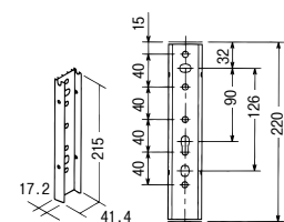
ベース取付座
