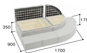
CUB-R60S 1セット+ CUB-8060W-3S 1セット
