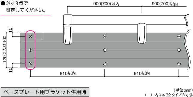
ベースプレート用ブラケット併用時 ( ) 内はφ32タイプの寸法
