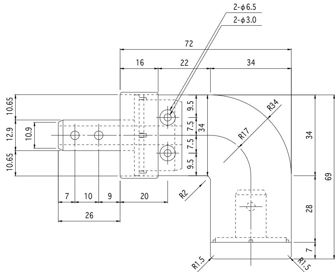
Z矢视图 (リベット詳細図)
