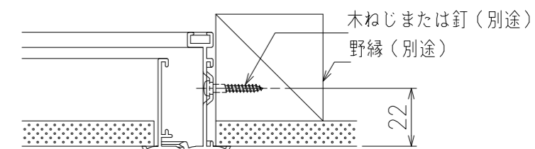
木製天井下地断面納まり図 (1:2)
