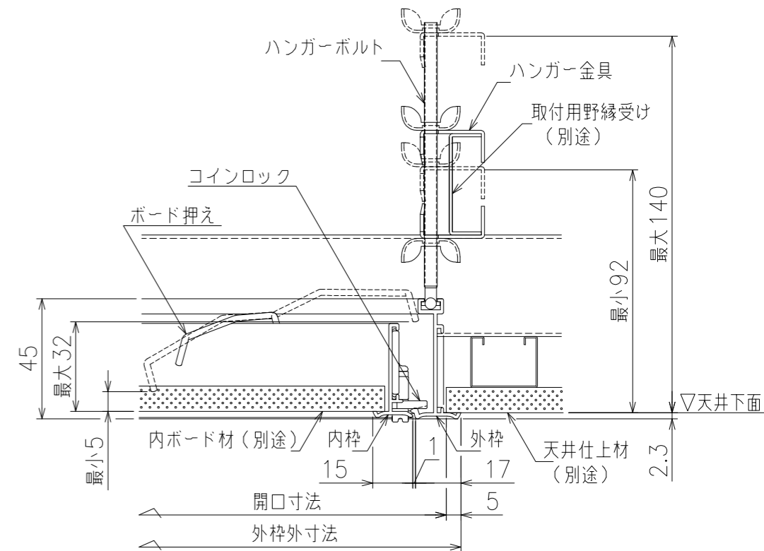
鋼製天井下地断面納まり図 (1:2)
