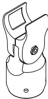
支柱用自在ジョイント (EZ-10US)
