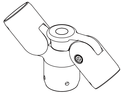
支柱用コーナージョイント (EZ-18US)
