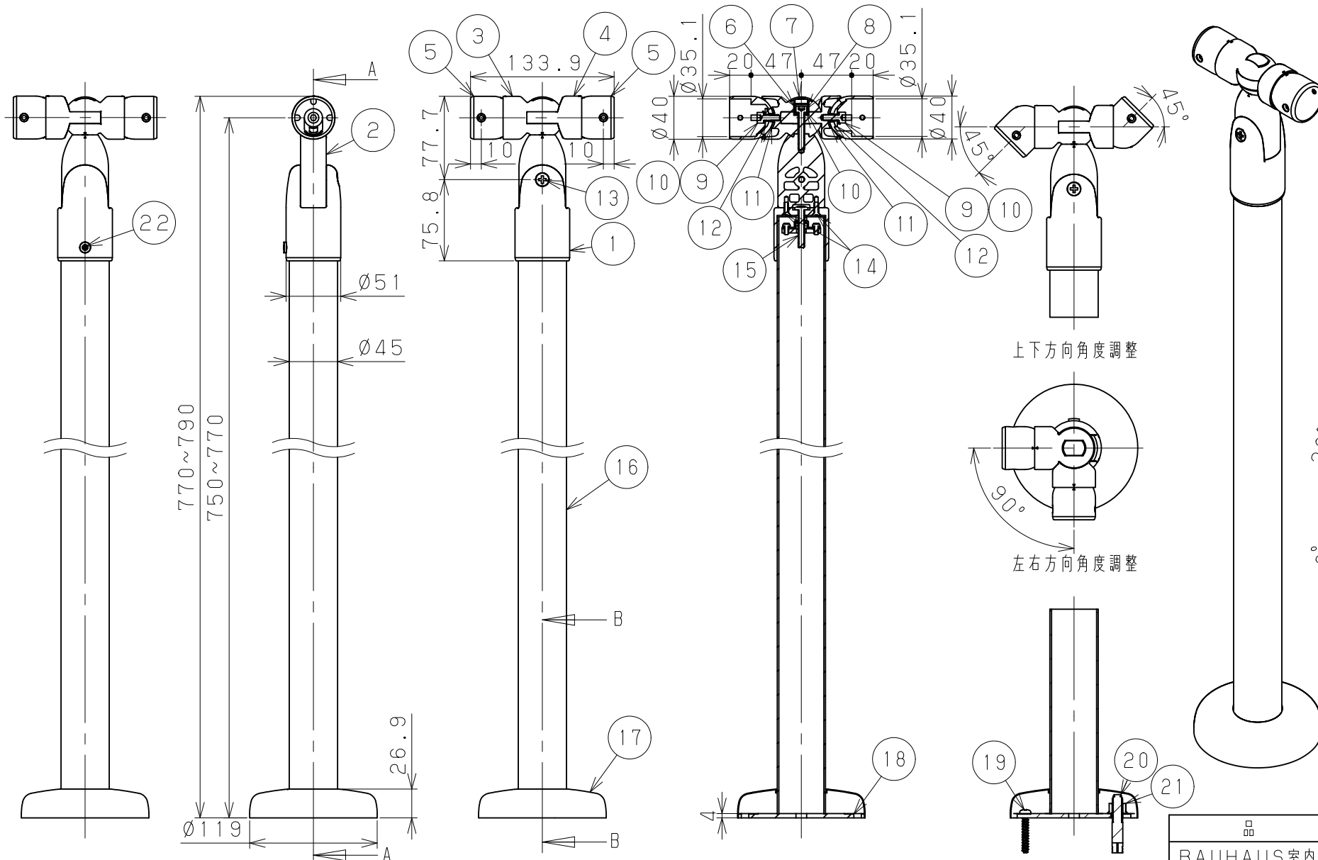
A-A section
